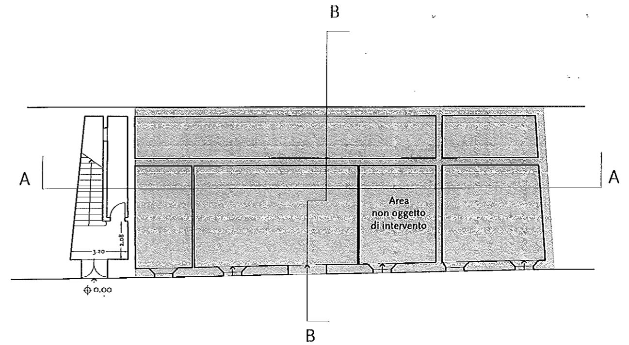
Pianta livello accesso da via Roma
