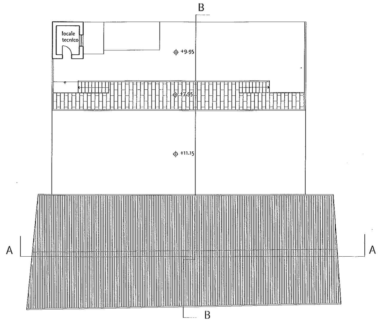
Pianta livello terrazza
