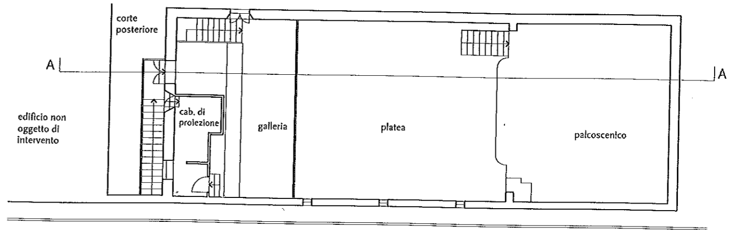
Pianta livello galleria
