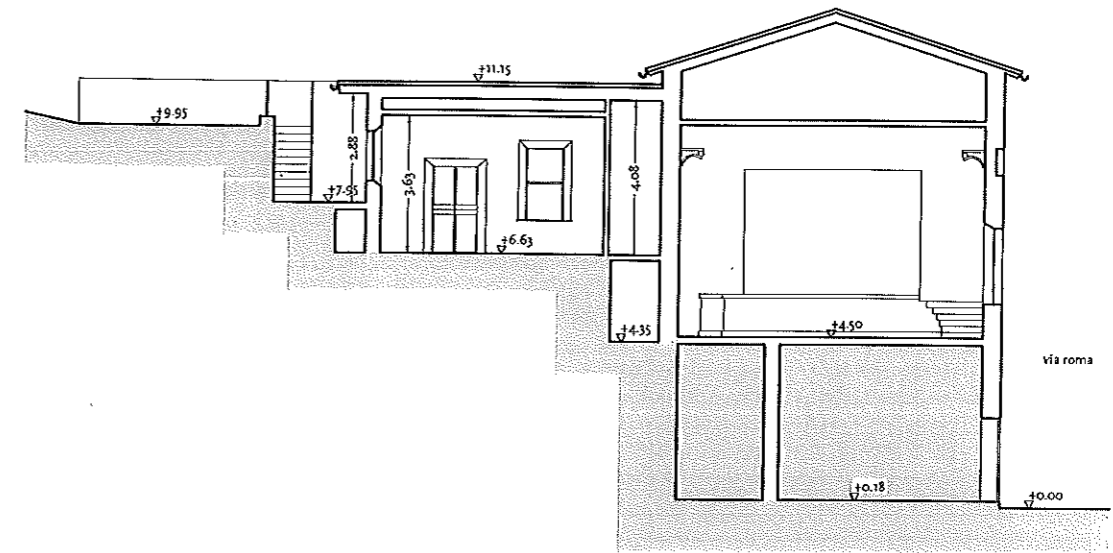
Sezione BB
