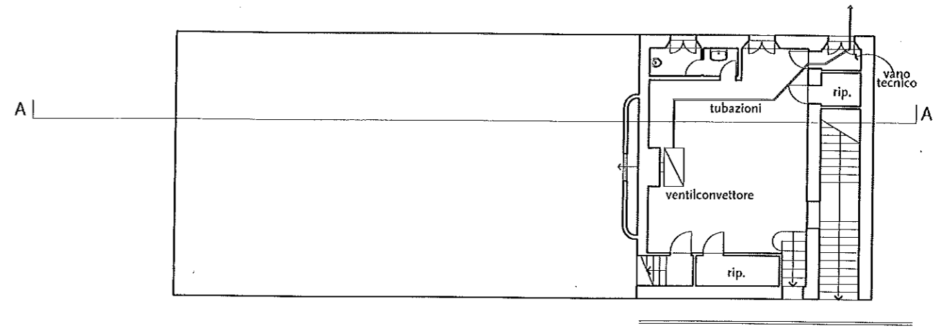
Pianta livello sottopalco
