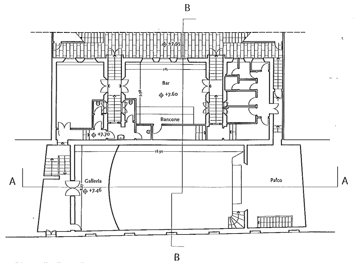
Pianta livello galleria
